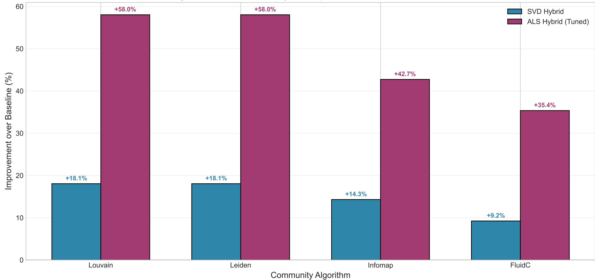
Figure 40: SVD and ALS Hybrid Improvement over Best Baseline
